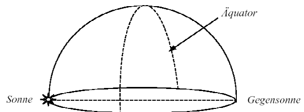
Abbildung 2: Halbsphäre des Himmels mit Polen und Äquator beim Sonnenuntergang.
