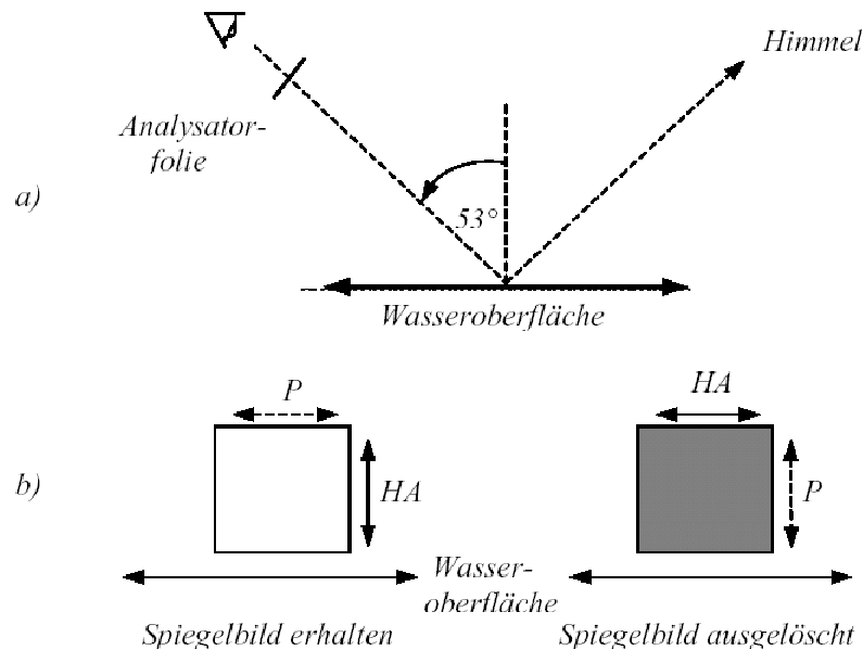
Abbildung 3: a): "Schrägblick" auf die Wasseroberfläche. b): Ansichten des hellen Himmels im Wasserspiegel durch eine Analysator-Folie mit horizontaler beziehungsweise vertikaler Polarisationsrichtung P, HA kennzeichnet die Hauptachsenlage der Folie.
