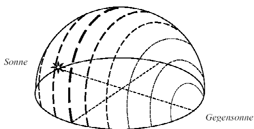
Abbildung 4: Halbsphäre des Himmels bei Sonnenuntergang mit Polarisationsrichtungen. Die Strichstärke entspricht dem relativen Polarisationsgrad.
