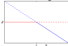
Bifurkationsdiagramm
